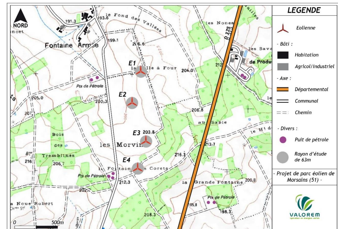
Zone d'effet du phénomène « Chute d'éléments de l'éolienne »
