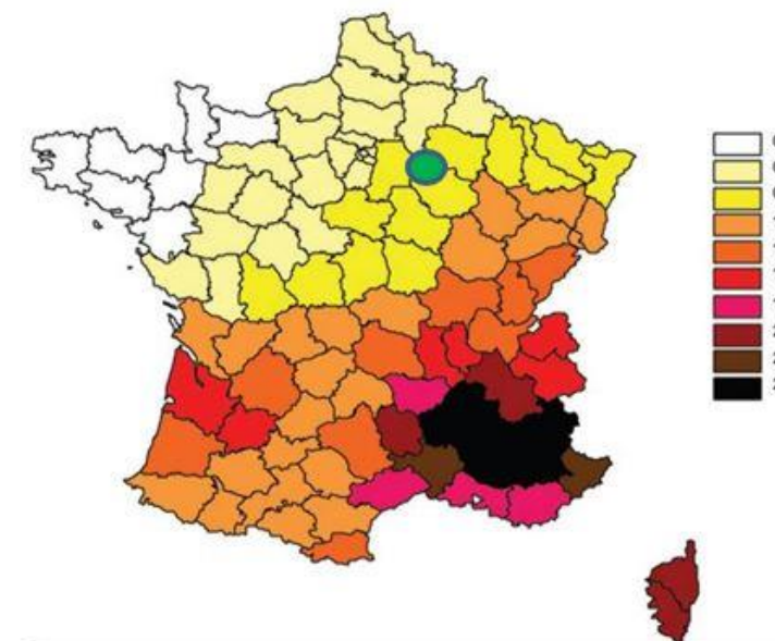
Répartition des impacts de foudre sur le territoire français métropolitain
