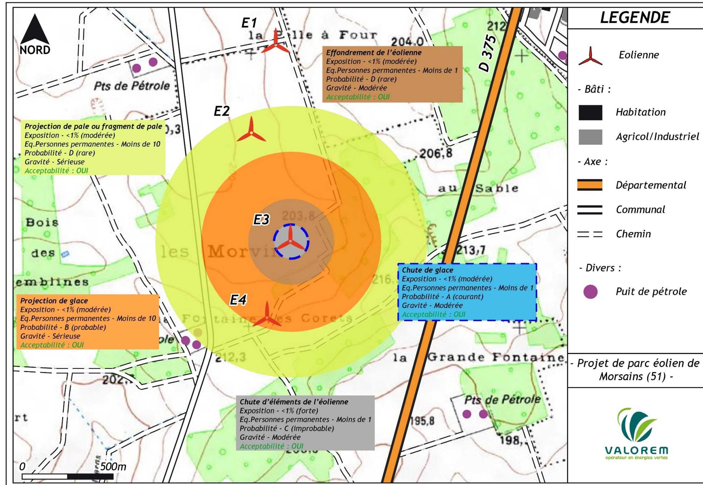
Synthèse des zones d'effet - éolienne E3
