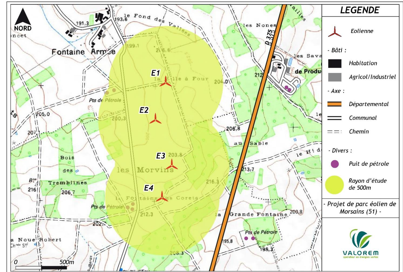
Zone d'effet du phénomène « Projection de pales ou de fragments de pales »
