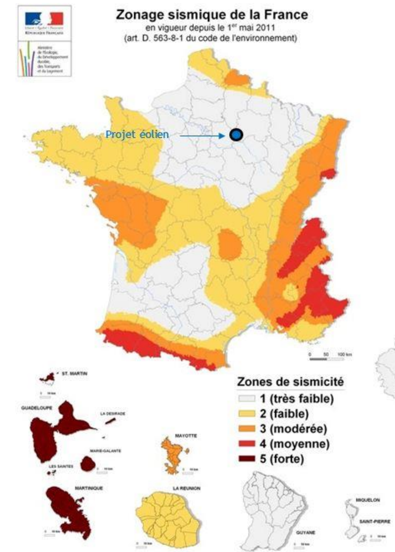
L'aléa sismicité en France et dans la région du site d'étude
